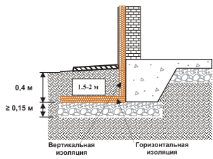
Рис. 1. Отапливаемое помещение
