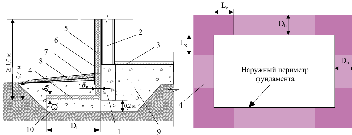
Рисунок 11.2. Схема укладки и параметры теплоизоляции в фундаментах отапливаемых зданий без теплоизоляции пола:
