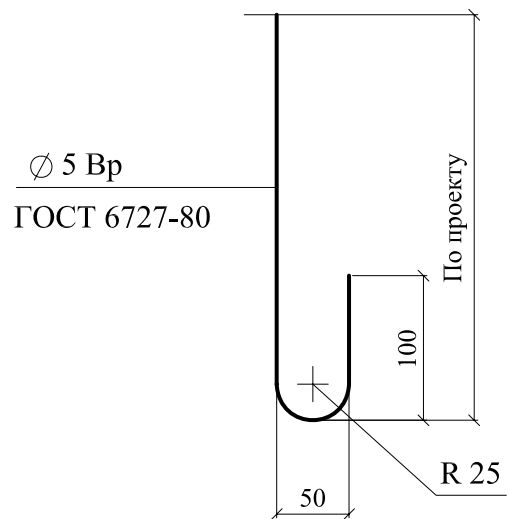
ЗАКЛАДНАЯ ПЕТЛЯ ЗП2
