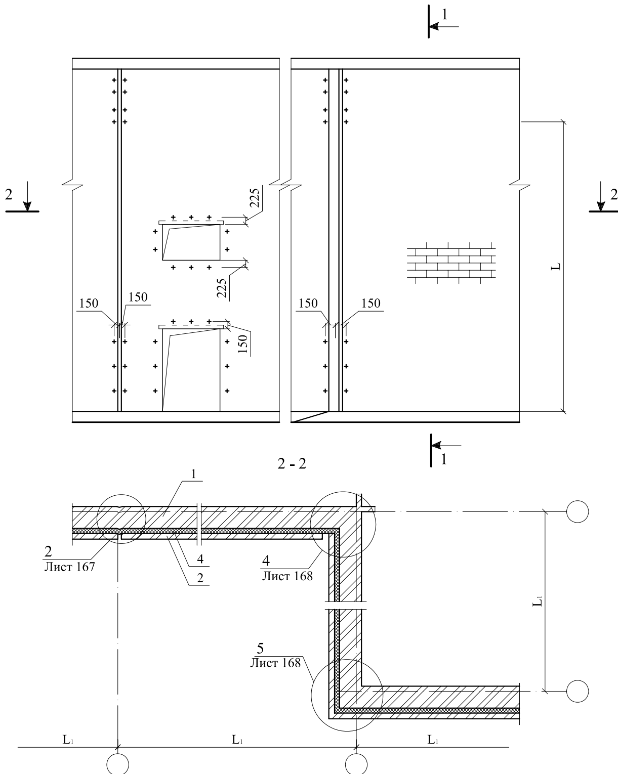
СХЕМА № 2. Расположение дюбелей в углах, температурных швах и у проемов
