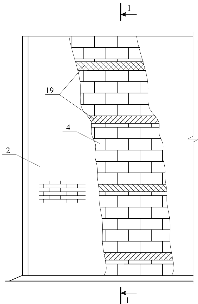
СХЕМА № 1. Расположение плит утеплителя, расщечек
