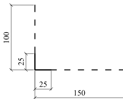
УГЛОВОЙ КОМБИНИРОВАННЫЙ ПРОФИЛЬ
