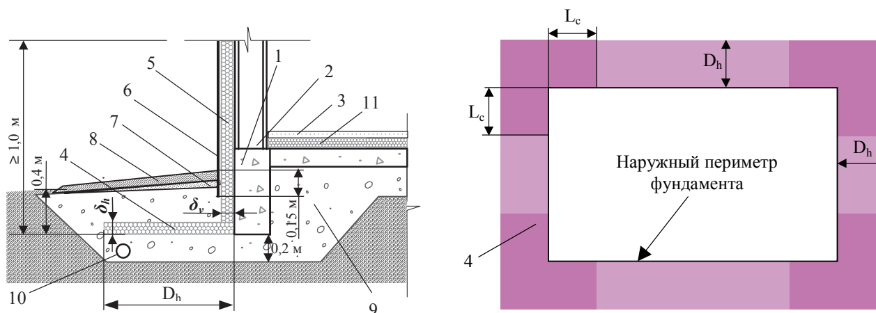
Рисунок 11.1. Схема укладки и параметры теплоизоляции в фундаментах отапливаемых зданий с теплоизоляцией пола:
