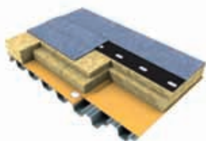
Система однослойной кровли по профлисту
