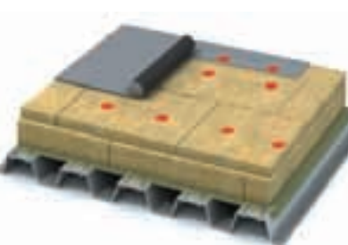
Система TN-классик
